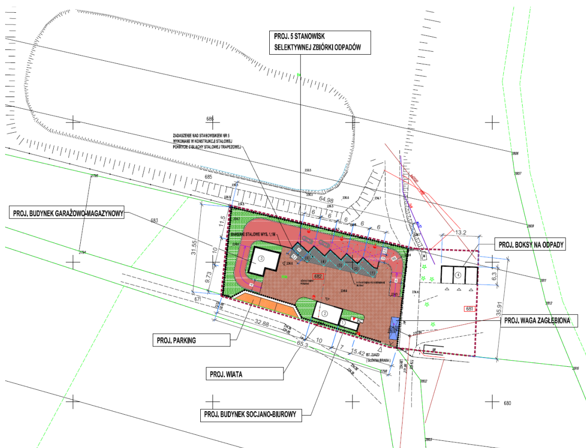
Rys.2. Projekt PSZOK
