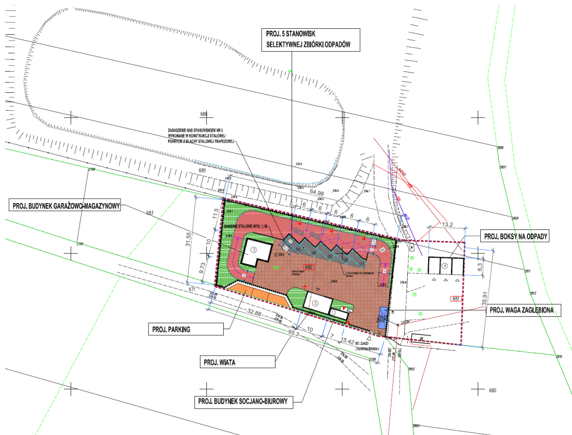
Rys.2. Projekt PSZOK
